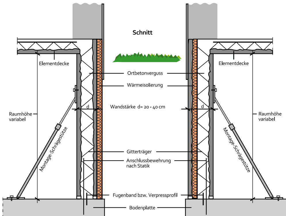
Hohlwand mit Außenwärmedämmung
